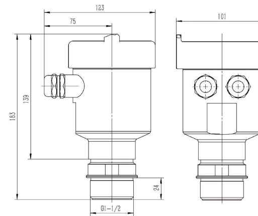
G1-1/2管螺纹过程连接常温结构尺寸示意图
