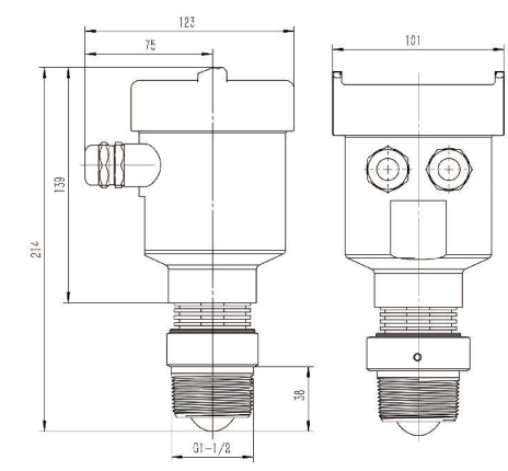
G1-1/2管螺纹过程连接高温结构尺寸示意图
