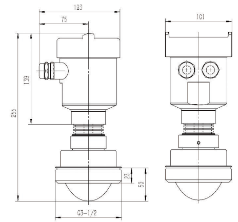
G3-1/2管螺纹过程连接高温结构尺寸示意图
