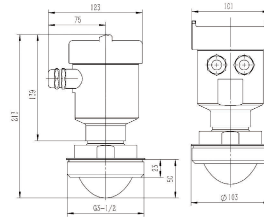
G3-1/2管螺纹过程连接常温结构尺寸示意图
