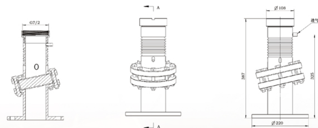
(1200℃高温法兰隔温装置示意图)
