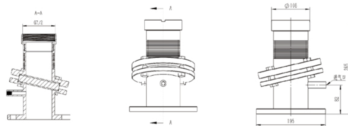
(350℃高温法兰隔温装置示意图)
